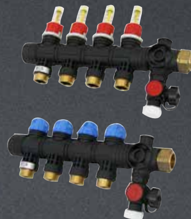
Roth Kunststoff Heizkreisverteiler mit DFA G1
